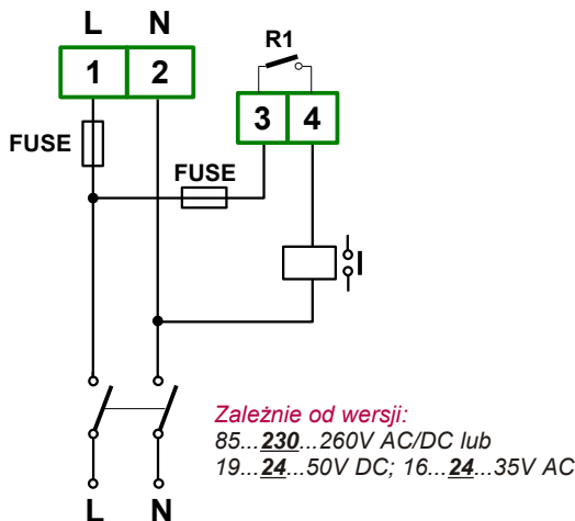
Rys. 4.7. Podłączenie zasilania oraz przekaźników sterujących obciążeniami
