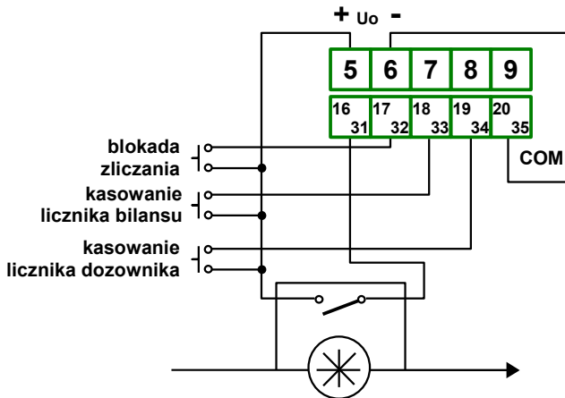
Rys. 4.16. Przykładowe podłączenie przetwornika przepływu z wyjściem kontaktorowym
