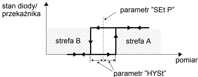
Rys. 6.3. Sterowanie jednoprogowe wyjścia przekaźnikowego/ diody LED
