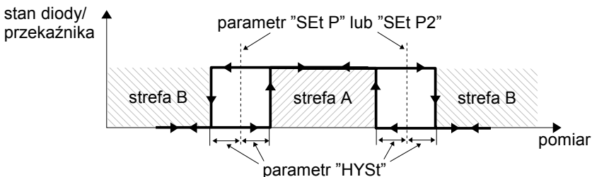
Rys. 6.4. Sterowanie dwuprogowe wyjścia przekaźnikowego/ diody LED
